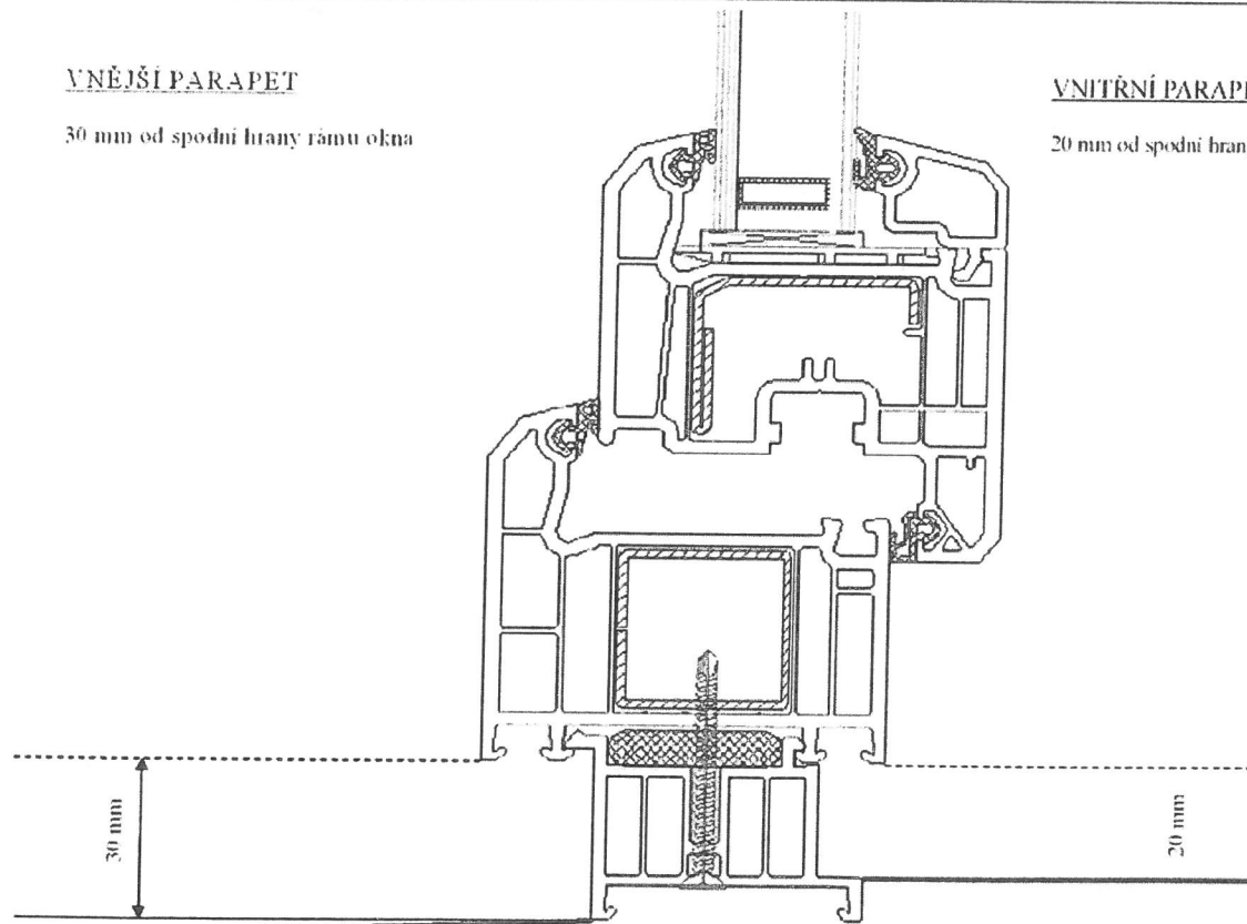
Betonové lůžko pro položení parapetů
